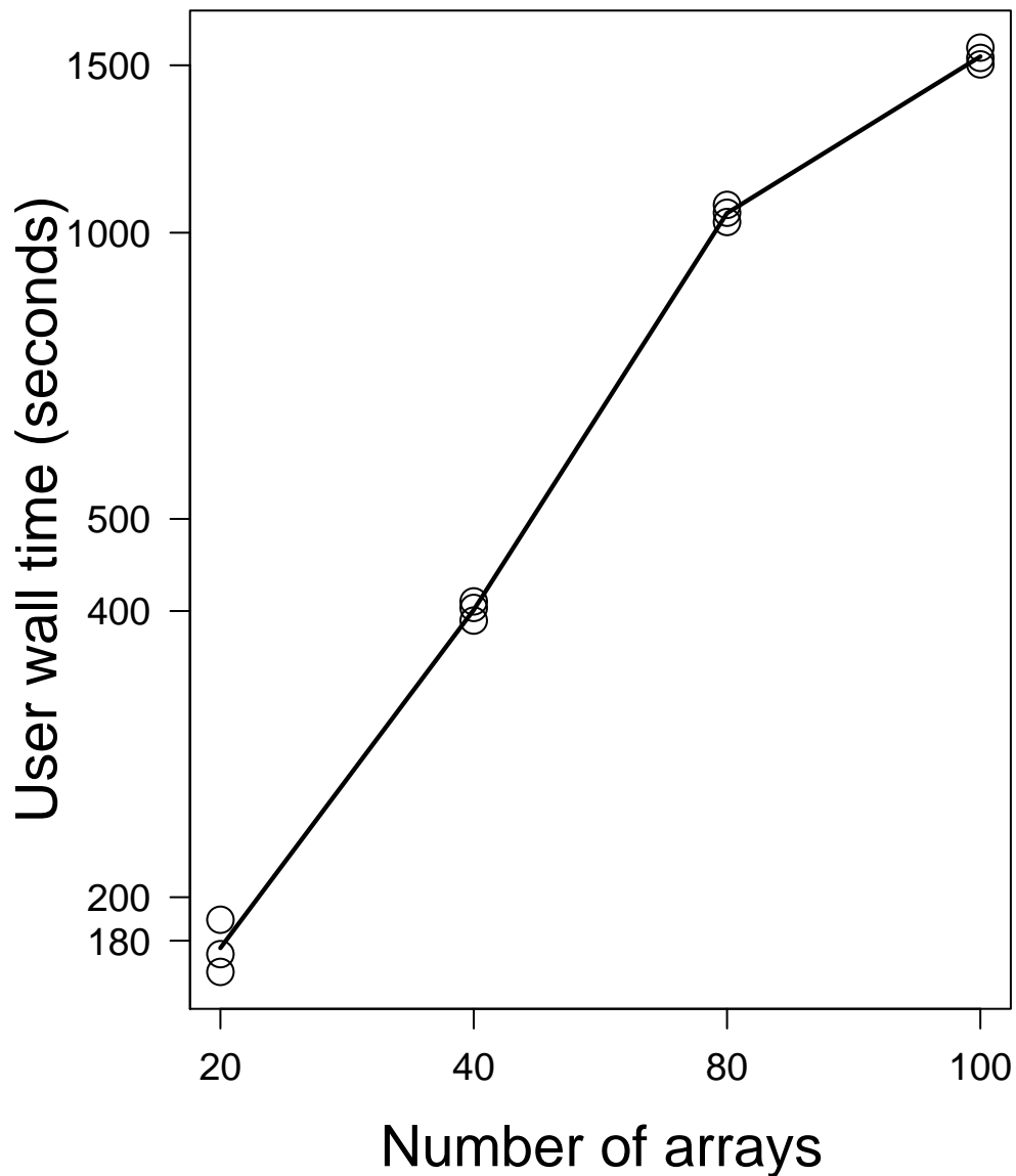
Prostate data set, 6033 genes
